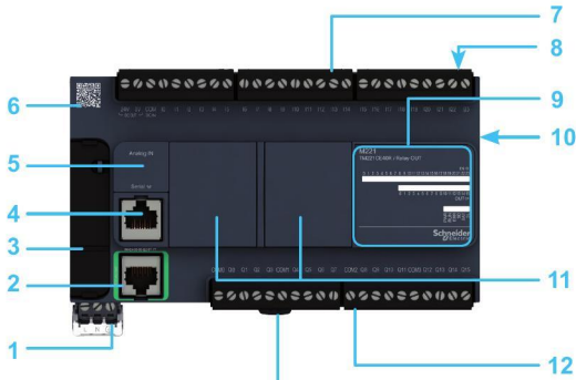
M221: 40 I/O
